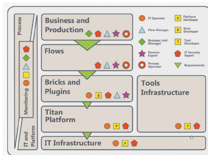
Titan Rollenmodell – Industrial DevOps Forschungsprojekt ( www.industrial-devops.org )
